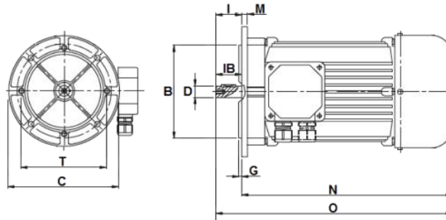
IEC - B5
